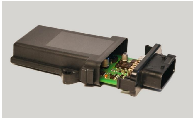
Abbildung 1: PEG-Fx 98-2: lange Variante mit 2 Anschraubpunkten (Leiterplatte nur als Beispiel)
