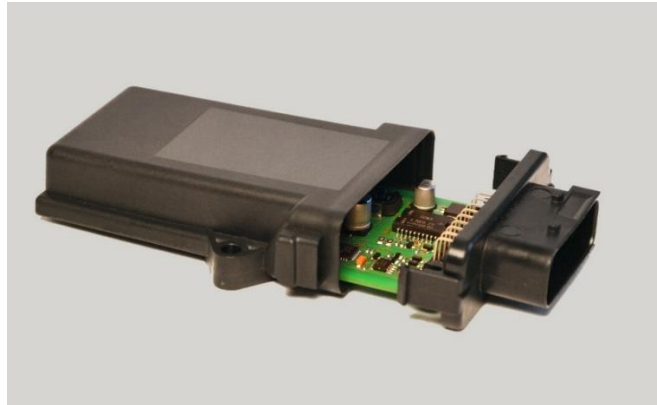
Abbildung 1: PEG-F 98-2: lange Variante mit 2 Anschraubpunkten (Leiterplatte nur als Beispiel)
